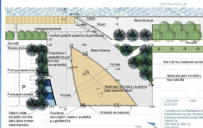
Laiva Toivon aukion yleissuunnitelma
